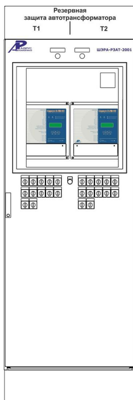
Шкаф резервных защит трансформатора и АУВ стороны ВН ШЭРА-РЗАТ-2001
